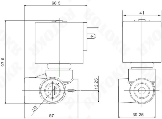
外形尺寸图
